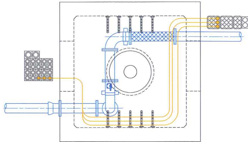
7-7 1段目フック
