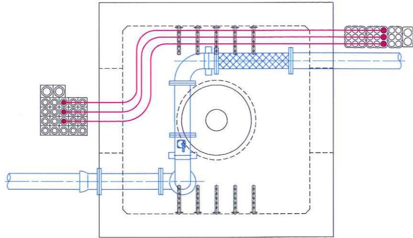
4-4 4段目フック
