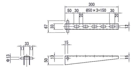
ケーブルフック S=1:5
